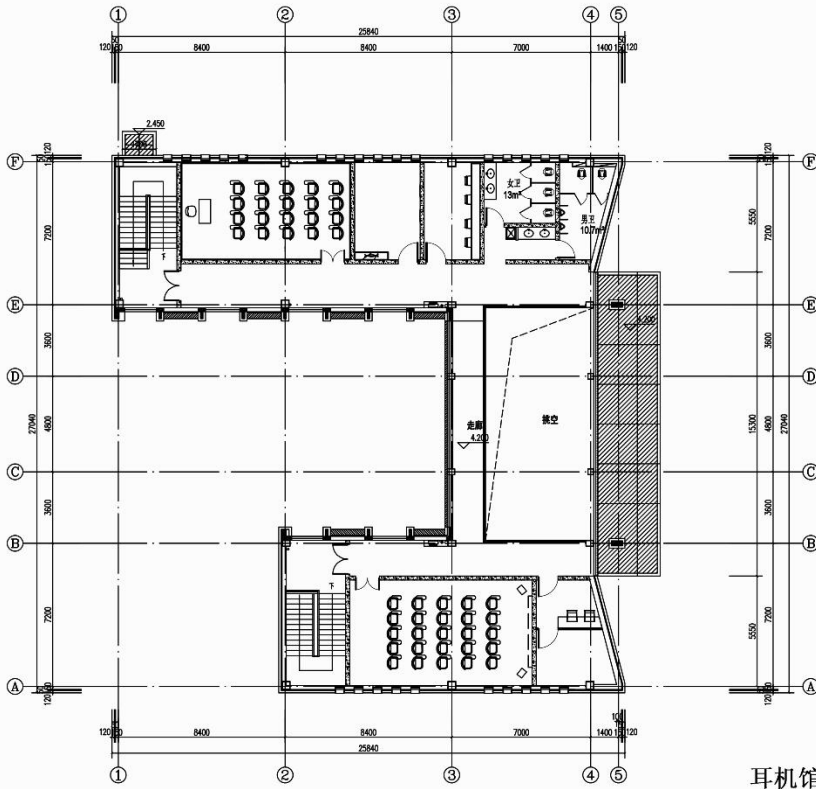
耳机馆二层平面图
